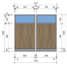
组合办公套装 (隔断) 侧立面图1: 20
