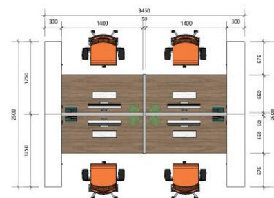
组合办公套装平面图1: 30
