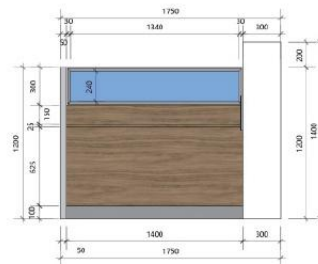
组合办公套装 (隔断) 正立面图1: 20
